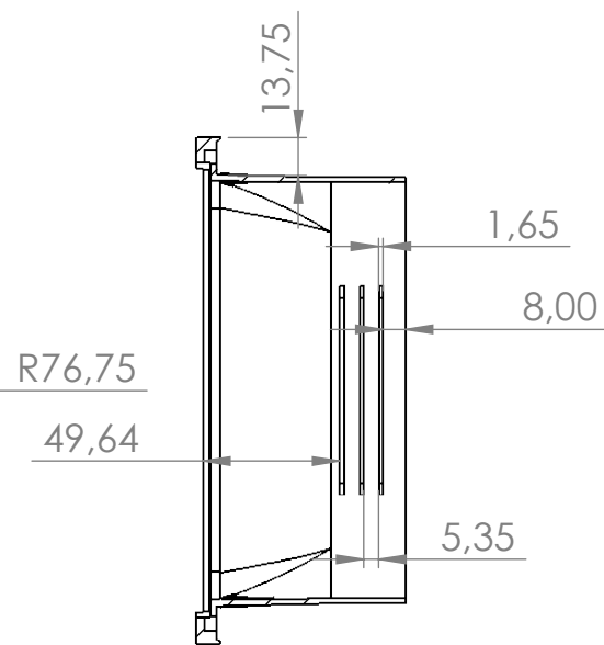
SEÇÃO A-A
